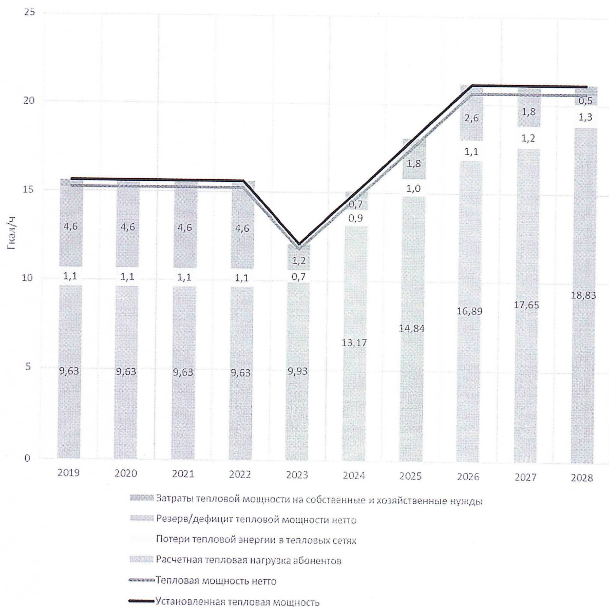
унок 7.1 – Балансы тепловой мощности и тепловой нагрузки в зоне действия котельной №5 (с 2023 года в зоне действия новой БМК)
