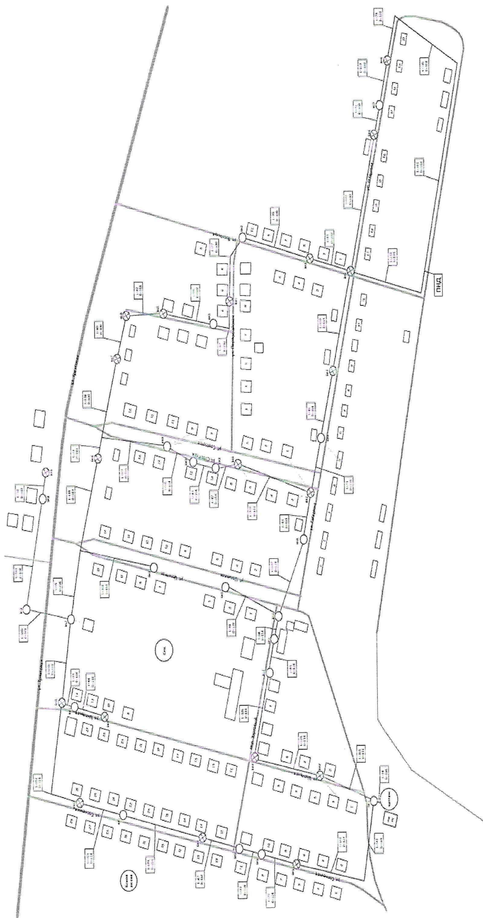
Рисунок 2. Схема водоснабжения сельского поселения Воротского сельсовета Ширинского муниципального района Республики Хакасия
